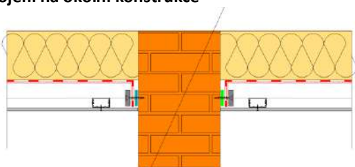
Napojení na zdivo butylovou oboustrannou páskou nebo Sunflex – pružným tmelem a přítlačnou lištou
