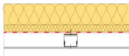
Napojení na dřevo butylovou oboustrannou páskou nebo Sunflex – pružným tmelem a přítlačnou lištou
